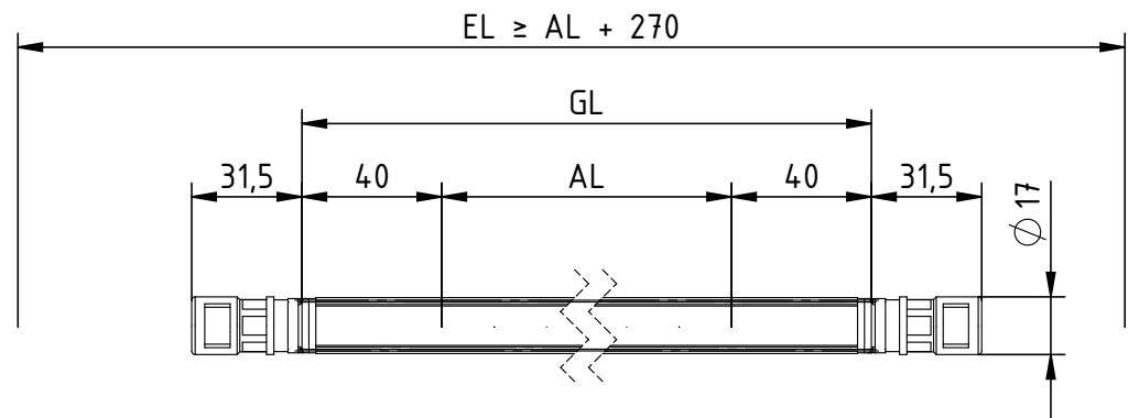
Abb. 15: Durchgangs- elektrode R51A/D mit zwei axialen Anschlüssen
