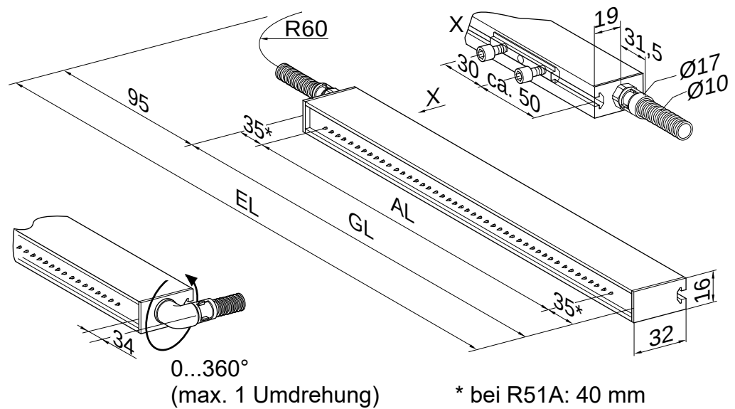
Abb. 13: Entladeelektrode R50 / R51A
