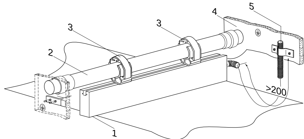
Abb. 5: Montage R50 mit GFK-Rundstab
