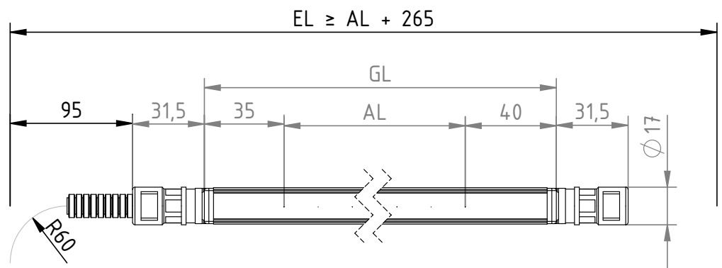
Abb. 14: Durchgangs- elektrode R50/D mit zusätzlichem axialen Anschluss
