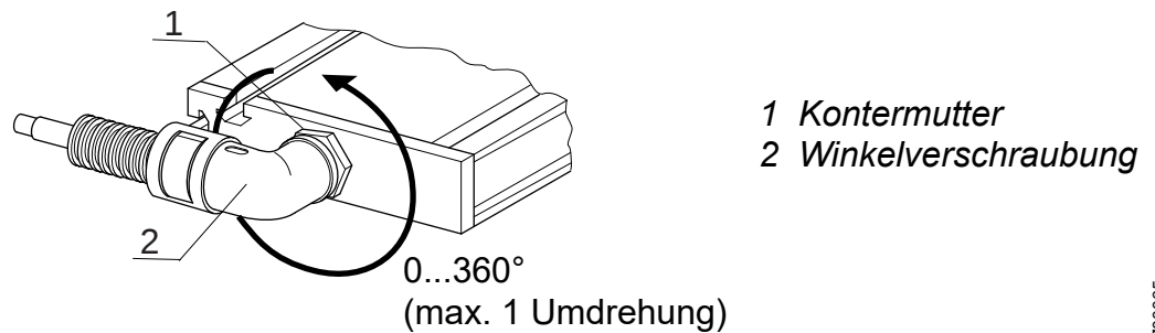
Abb. 6: Winkel- verschraubung
