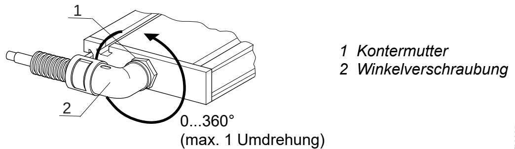
Abb. 6: Winkel- verschraubung
