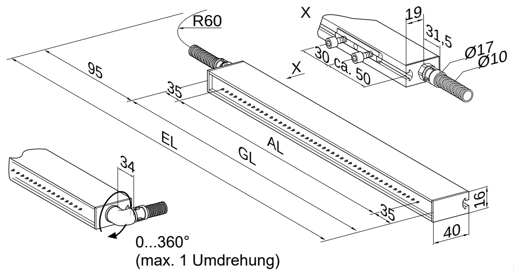
Abb. 7: Maßzeichnung Elektrode
