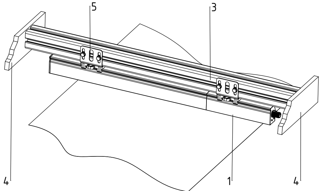
Abb. 5: Montagebeispiel SDS mit Stahlwin- kel und Alu-Profil
