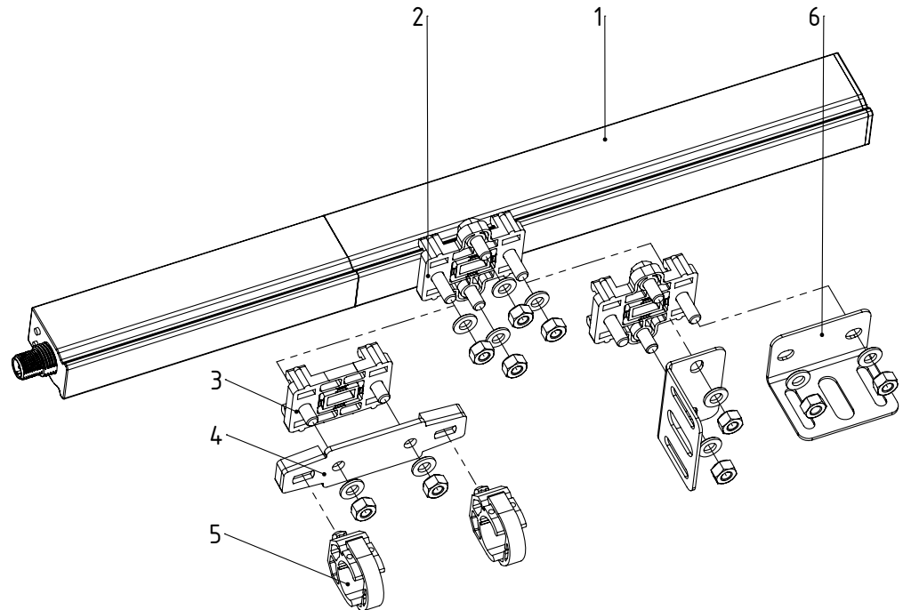
Abb. 4: Montage der Entladeelektrode SDS
