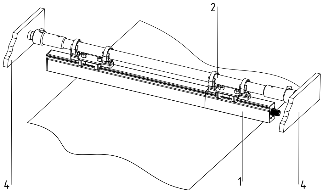
Abb. 6: Montage SDS mit GFK-Rundstab
