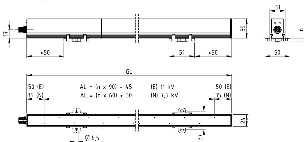
Abb. 2: Entladeelektrode SDS
