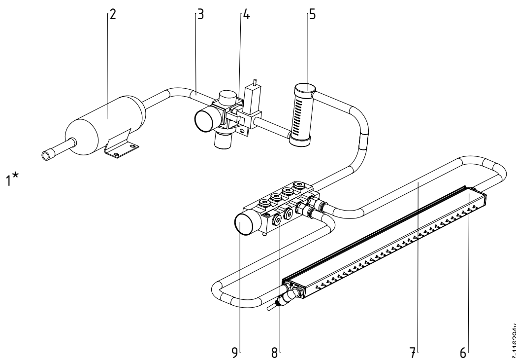
Abb. 9: Installation der Druckluftversor- gung
