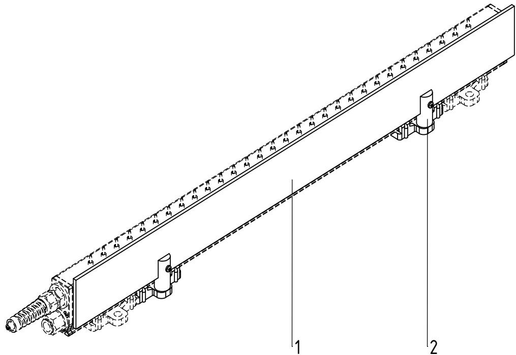
Abb. 6: Schutzprofil SP
