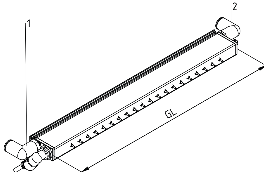
Abb. 8: Lage der Luftanschlüsse in Abhängigkeit von der Gesamtlänge GL
