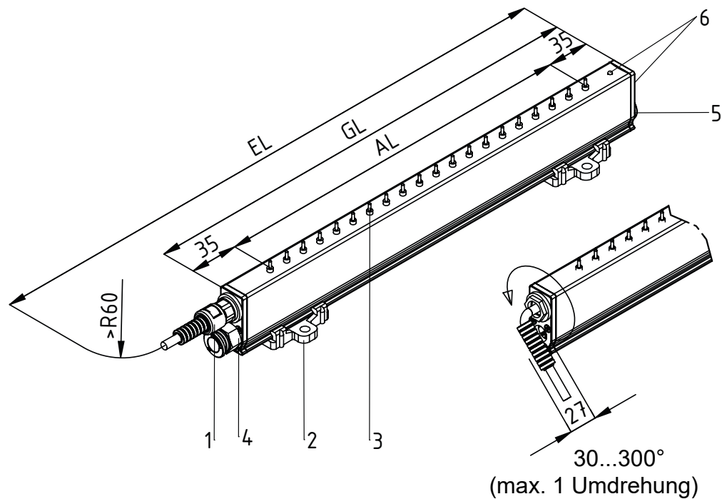
Abb. 1: Übersicht Entladeelektrode R60L
