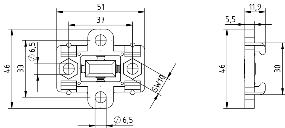
Abb. 13: Halter - Standard
