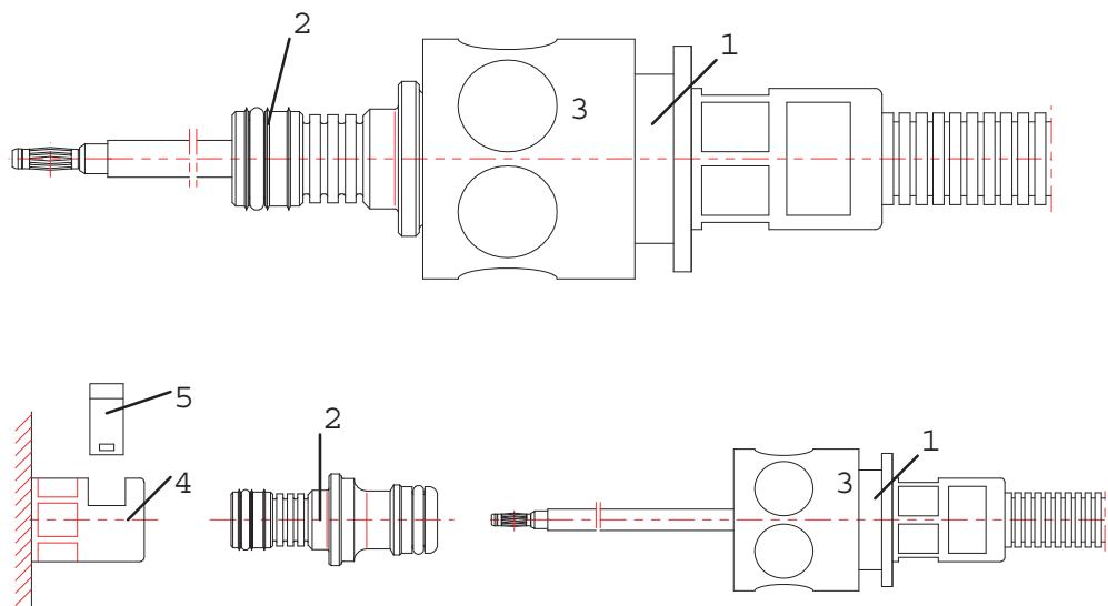
Abb. 12: Schnellsteckver- bindung für Aufla- dekomponenten
