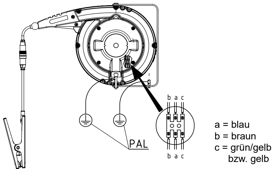
Abb. 9: Anschluss der Kabelrücklaufrolle 601KR/AW
