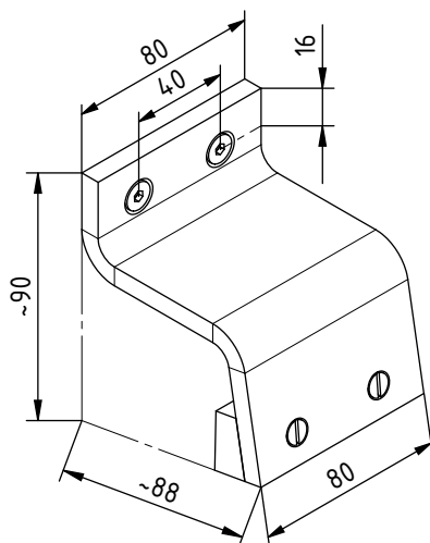
Abb. 18: Zangenhalter Artikel-Nr. 113112
