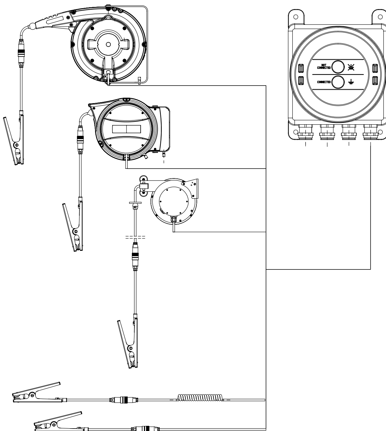
Abb. 1: Übersicht Erdüberwachungssystem TCB040-V2 mit Kabelrücklaufrollen und Zangen
