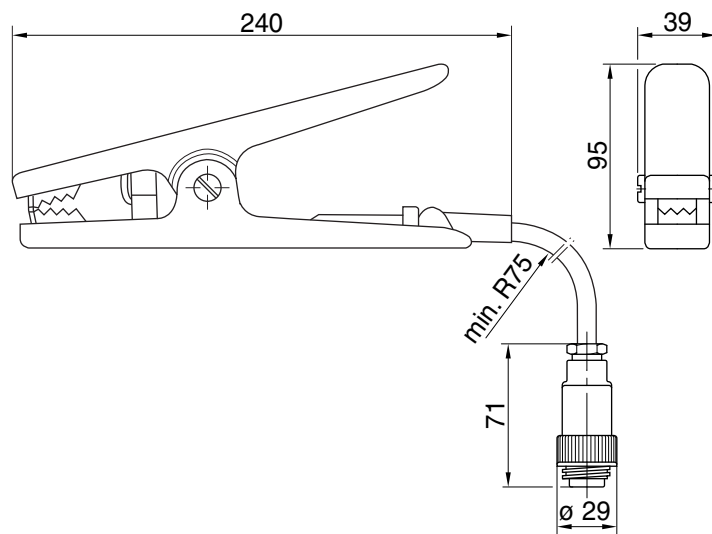
Abb. 20: Typ 70CG mit Kupplungsstecker; maximale Zangen- öffnung 35 mm
