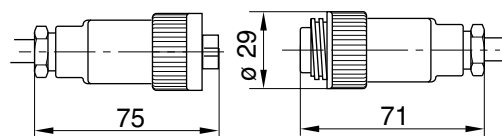
Abb. 22: Kupplungs- stecker / -buchse
