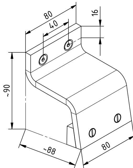
Abb. 24: Zangenhalter Artikel-Nr. 113112
