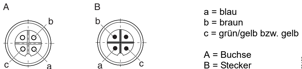
Abb. 14: Pinbelegung des Kupplungs- steckers
