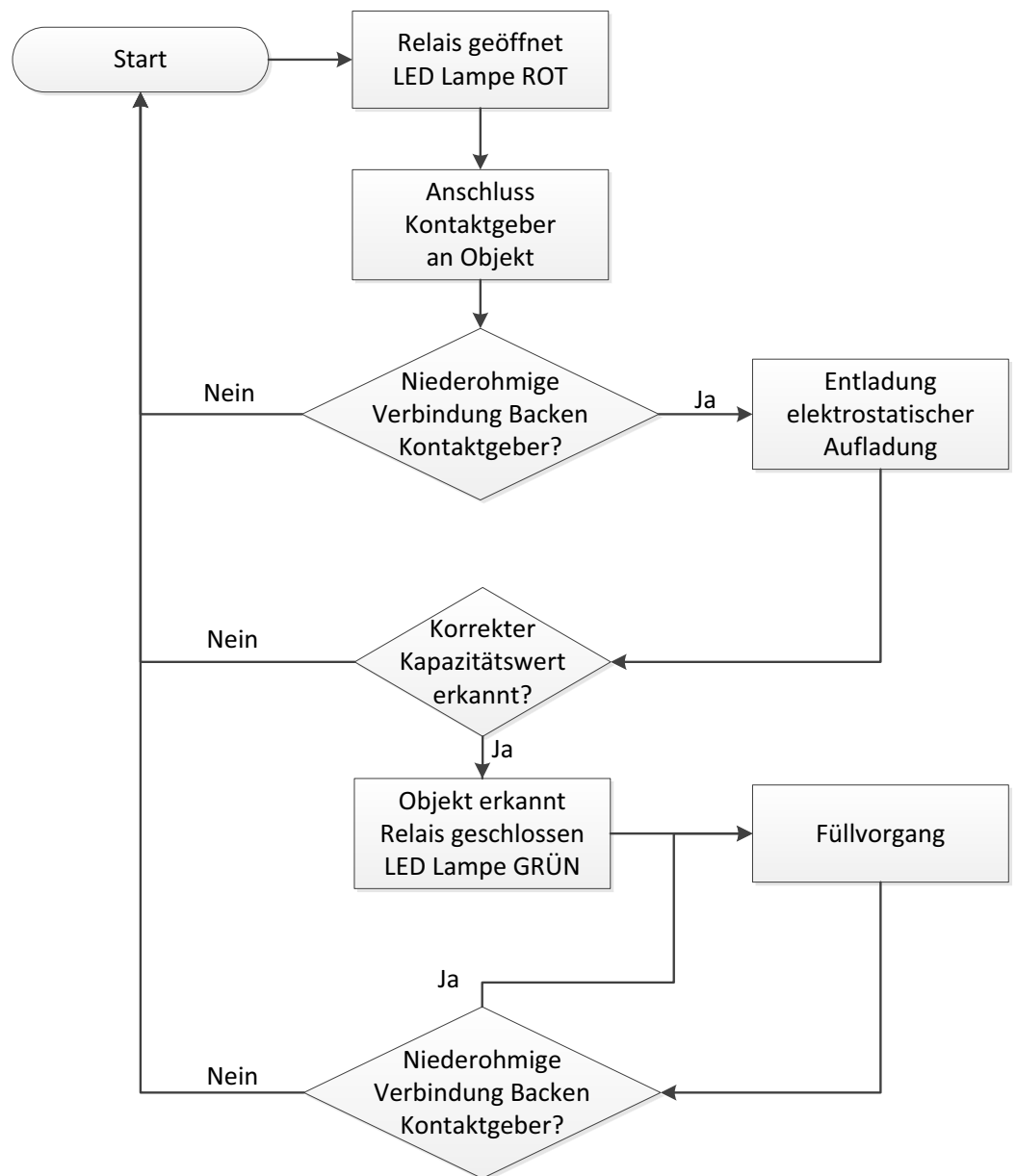
Abb. 2: Funktionsprinzip
