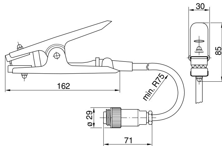
Abb. 21: Typ 70CK mit Kupplungsstecker; maximale Zangen- öffnung 35 mm
