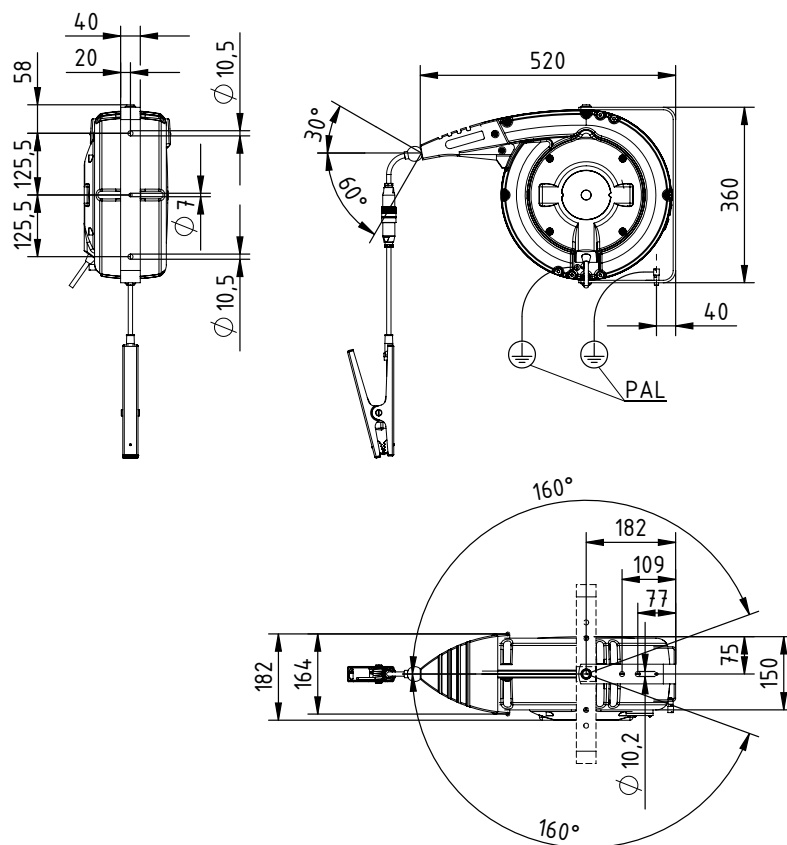
Abb. 25: Kabelrücklaufrolle Aluminium Typ 601KR/AW
