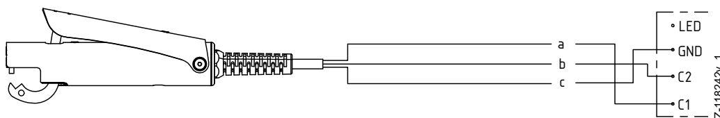
Abb. 11: Anschlussbeispiel Erdkontaktgeber TERRA-L
