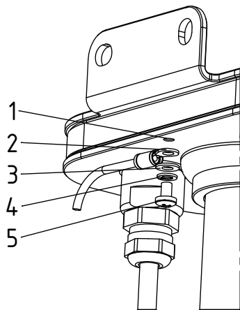
Abb. 5: Erdungsanschluss
