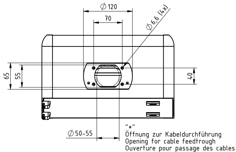
Abb. 54: Lochbild des Neigungsadapters ECC/NH und ECC/NI
