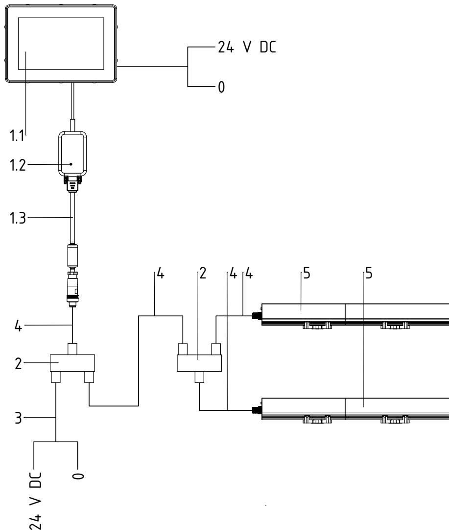
Abb. 4: Anbindungs- beispiel: Entladeelektrode SDS
