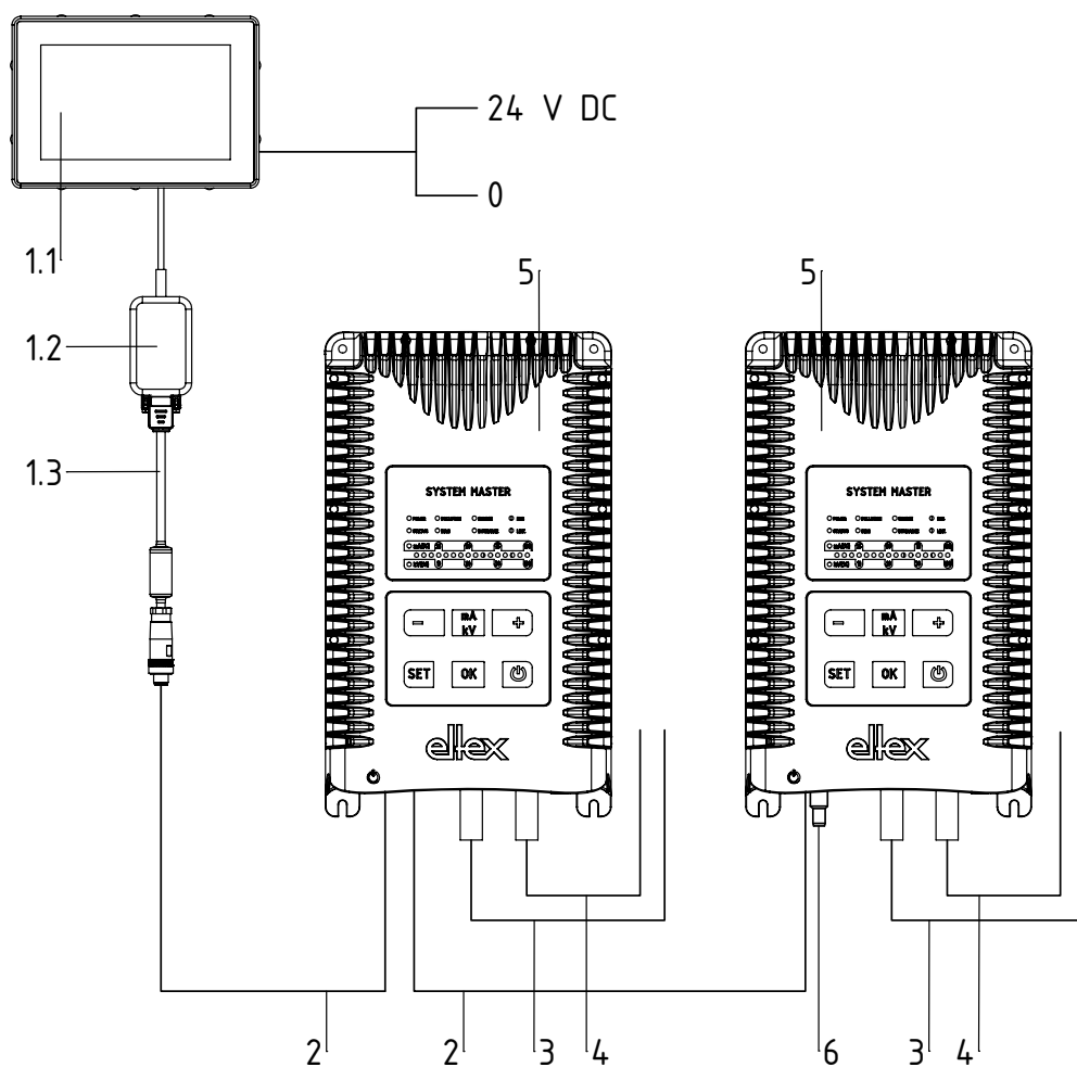
Abb. 3: Anbindungs- beispiel: Aufladegenerator POWER CHARGER PC
