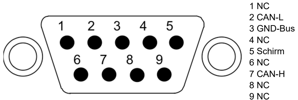
Abb. 1: Steckerbelegung D-Sub Steckverbinder
