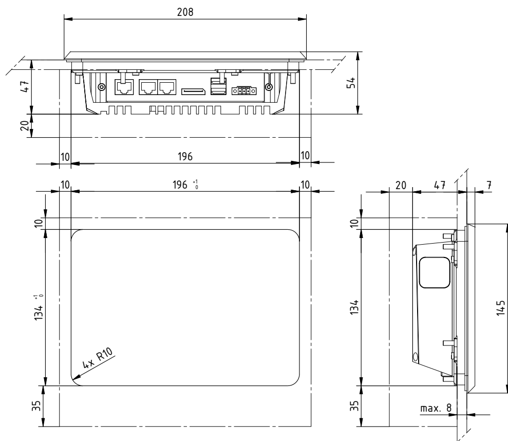
Abb. 41: Einbauausschnitt und Maße, Fernbedienung ECC/EK
