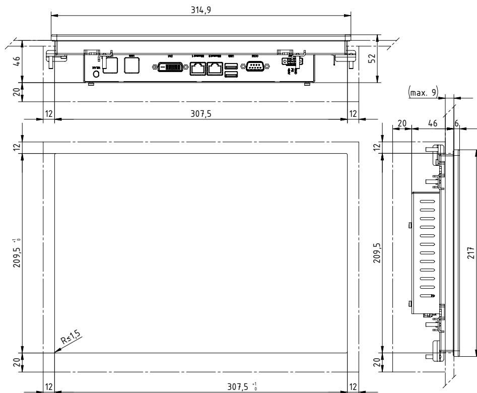
Abb. 43: Einbauausschnitt und Maße, Fernbedienung ECC/EH
