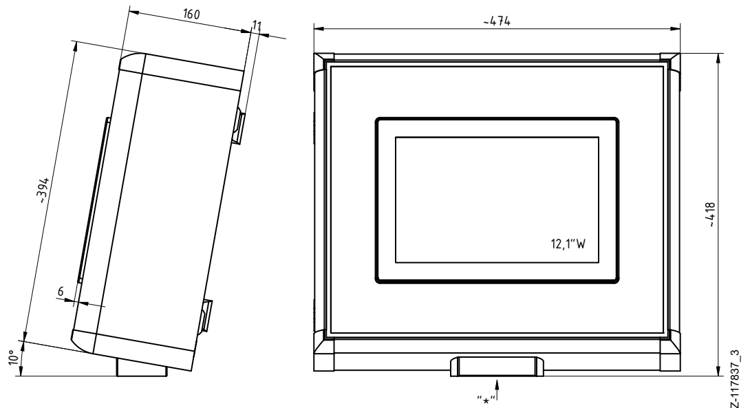
Abb. 53: Maße, Fernbedienung ECC/NH und ECC/NI
