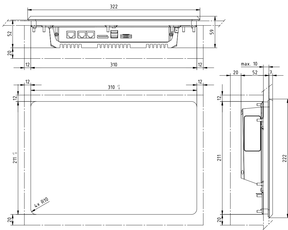
Abb. 45: Einbauausschnitt und Maße, Fernbedienung ECC/EI
