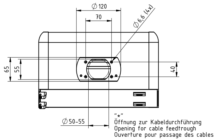
Abb. 52: Lochbild des Neigungsadapters ECC/NG und ECC/NK
