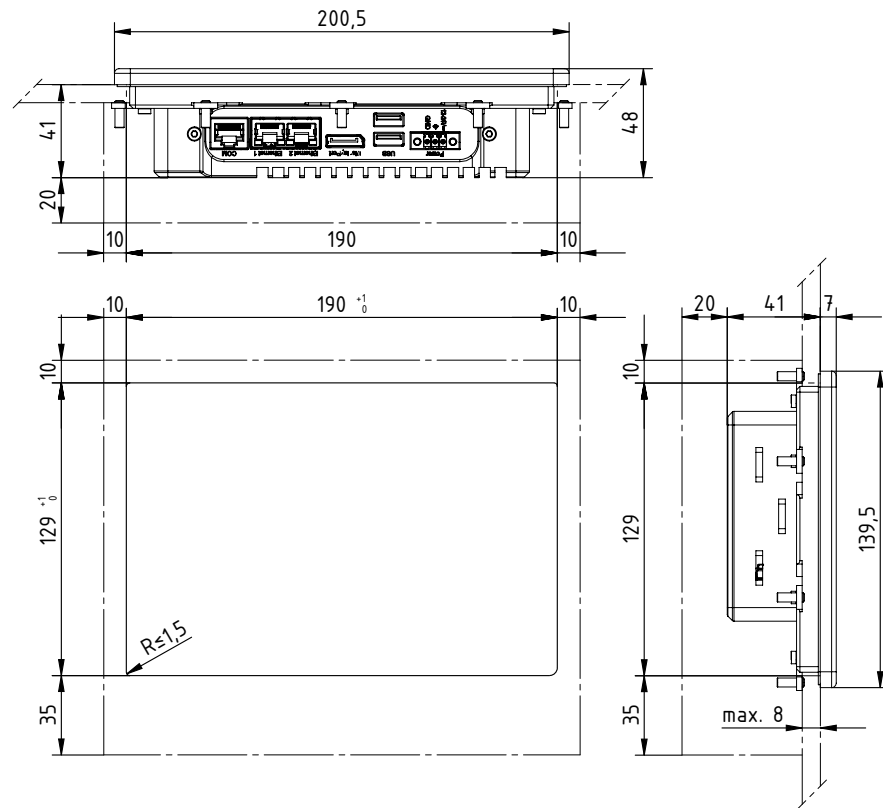
Abb. 39: Einbauausschnitt und Maße, Fernbedienung ECC/EG
