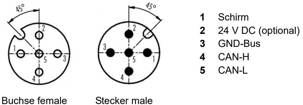
Abb. 2: Steckerbelegung M12-Rundsteck- verbinder
