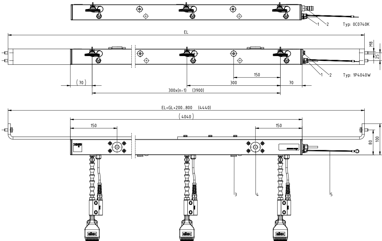
Fig. 13: Dimensions LR36 ion blower bar
