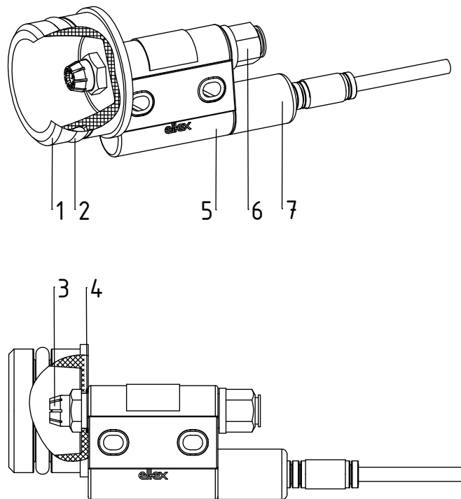
Fig. 4: EAR36E Discharge adapter
