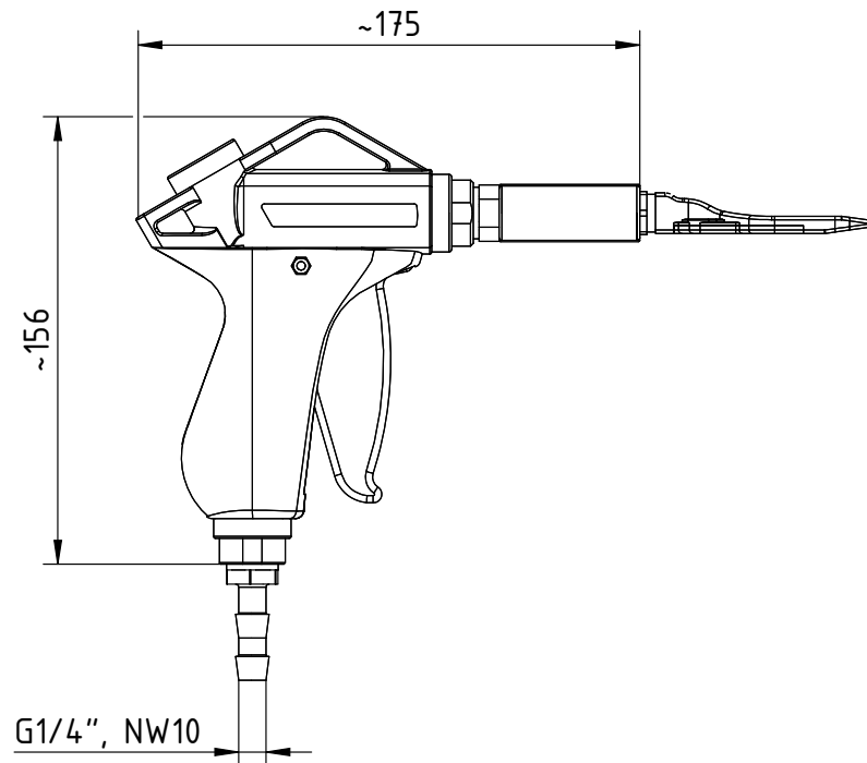
Fig. 14: Dimensions PR36/NF ion blower pistol
