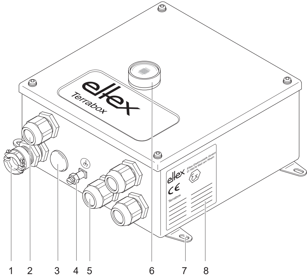
Fig. 2: Terrabox TCB030
