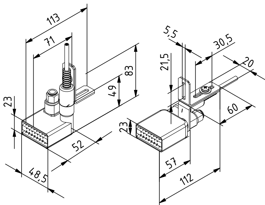
Fig. 3: Tête soufflante de décharge R55E, versions à raccords radiaux et axiaux avec fixation standard
