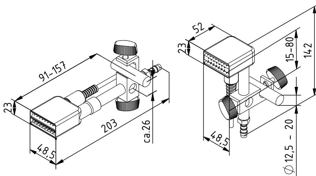
Fig. 4: Tête soufflante de décharge R55E, versions à raccords radiaux et axiaux avec fixation universelle
