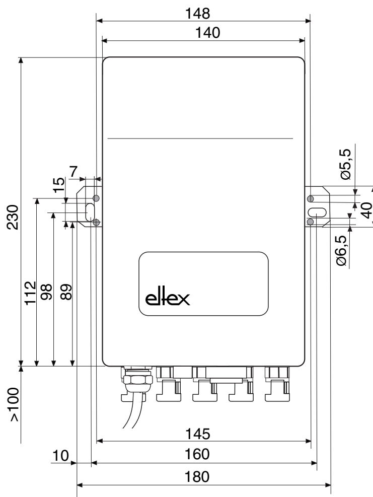
Fig. 2: Dimensions ES53
