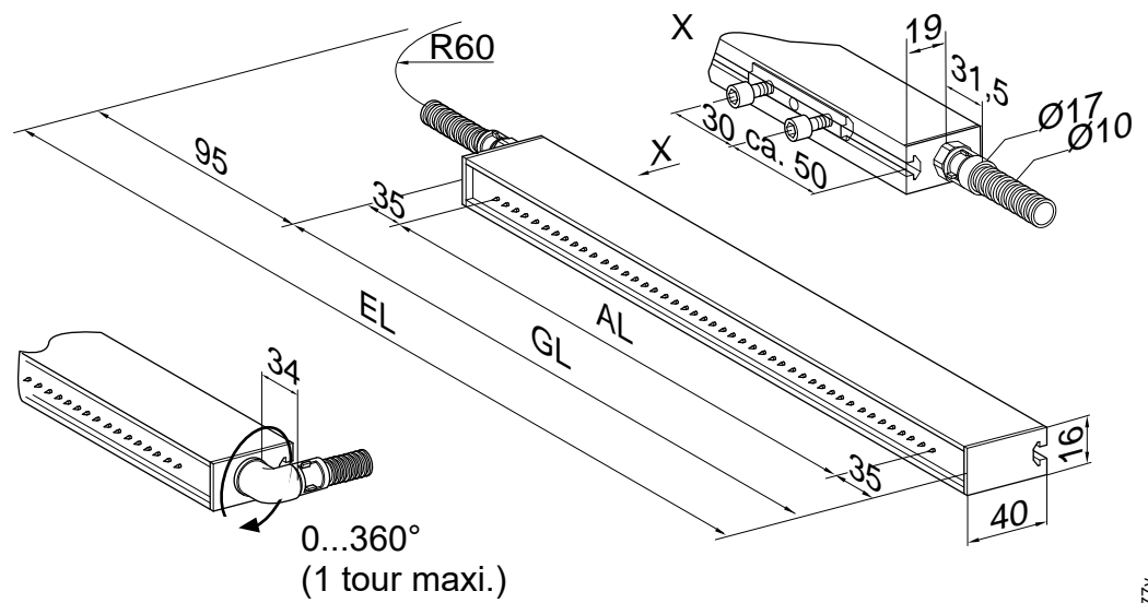
Fig. 8: Dimensions de l'électrode
