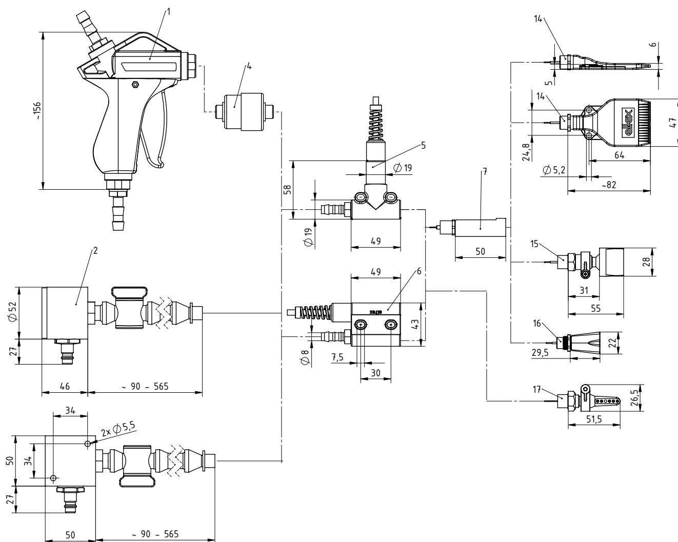
Fig. 12: Numéro de dessin Z-116969ey_2 Dimensions du pistolet soufflant de décharge, différentes buses et accessoires
