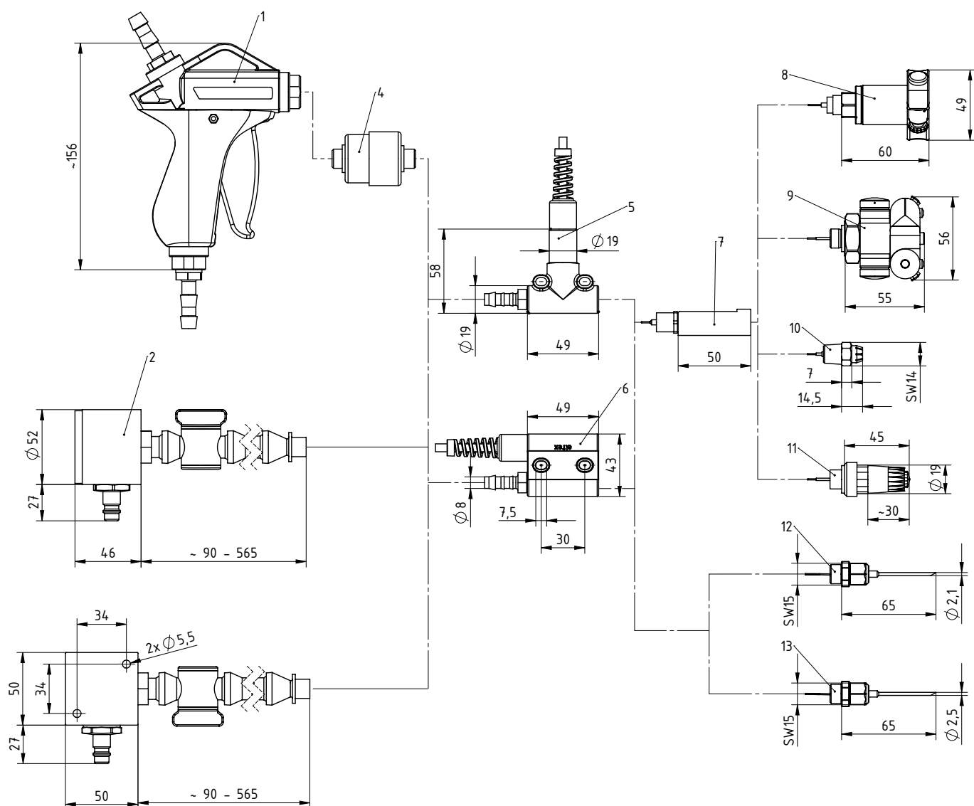
Fig. 11: Numéro de dessin Z-116969ey_1 Dimensions du pistolet soufflant de décharge, différentes buses et accessoires
