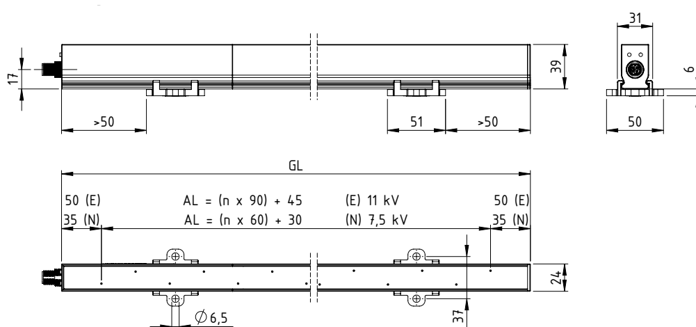
Fig. 2: Électrode de déc- harge SDS
