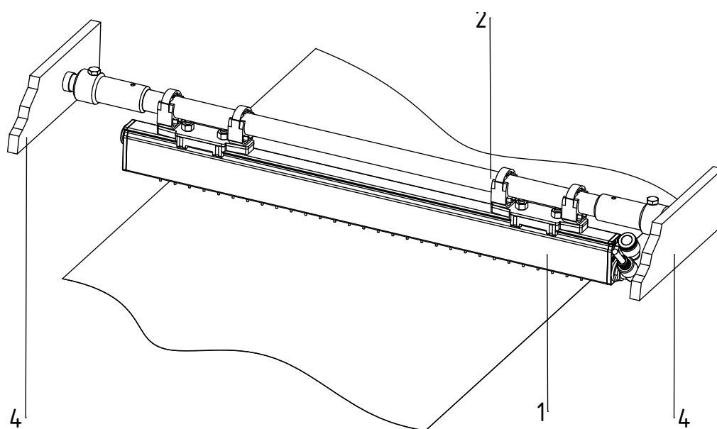
Fig. 6: Montage de SDS avec la barre ronde en plastique renforcé par fibres de verre
