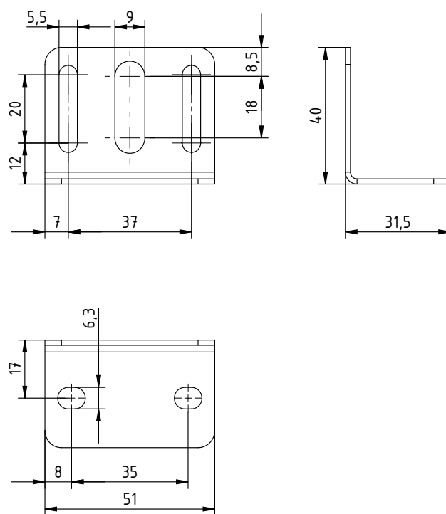
Fig. 12: Équiere de fixation
