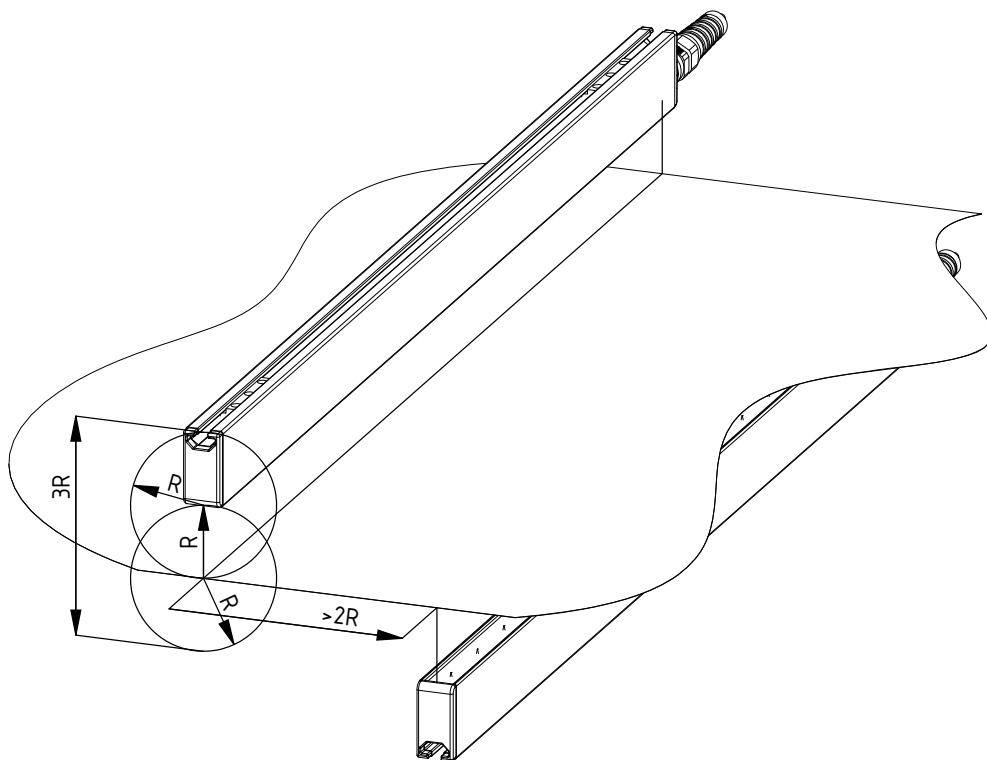
Fig. 5: Zone exempte de matériau conduc- teur avec les dimensions R
