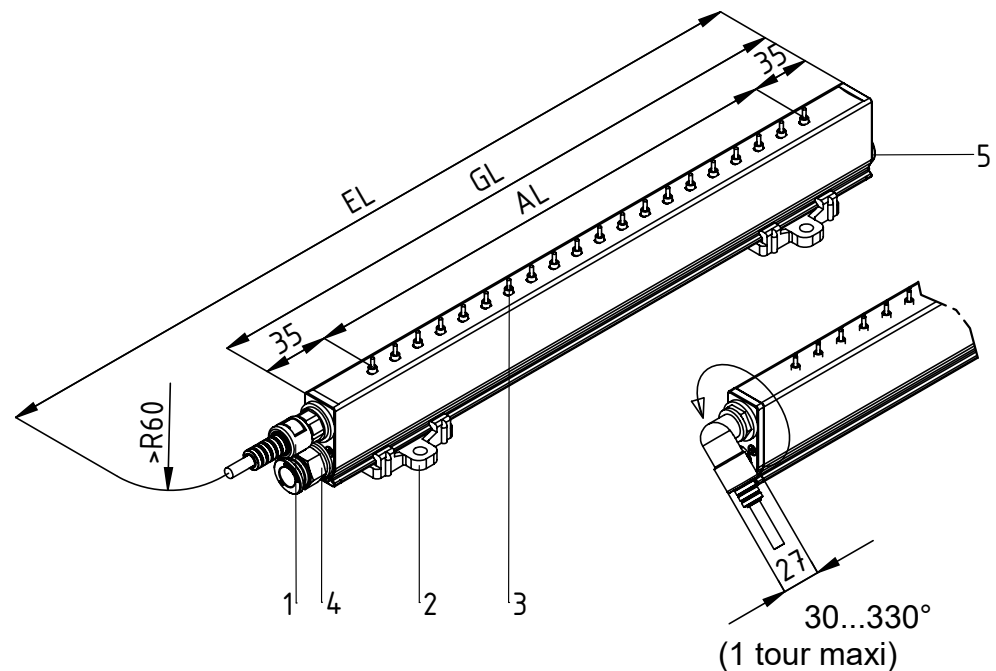
Fig. 1: Vue d'ensemble de l'électrode de décharge R60L
