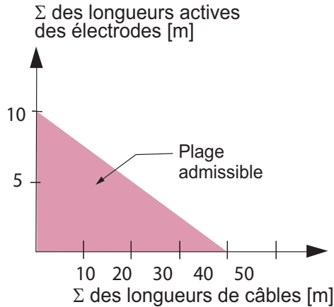
Fig. 7: Charge possible des alimentations PI, ES51 et ES60 en fonction de la longueur active de l'électrode et de la longueur du câble de haute tension
