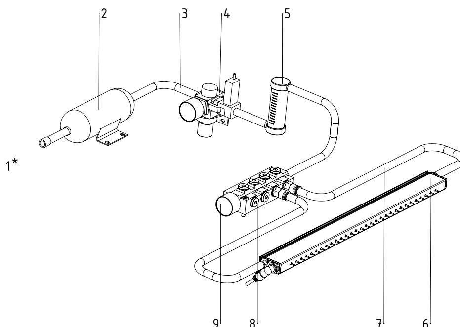
Fig. 12: Installation du système d'alimentation en air
