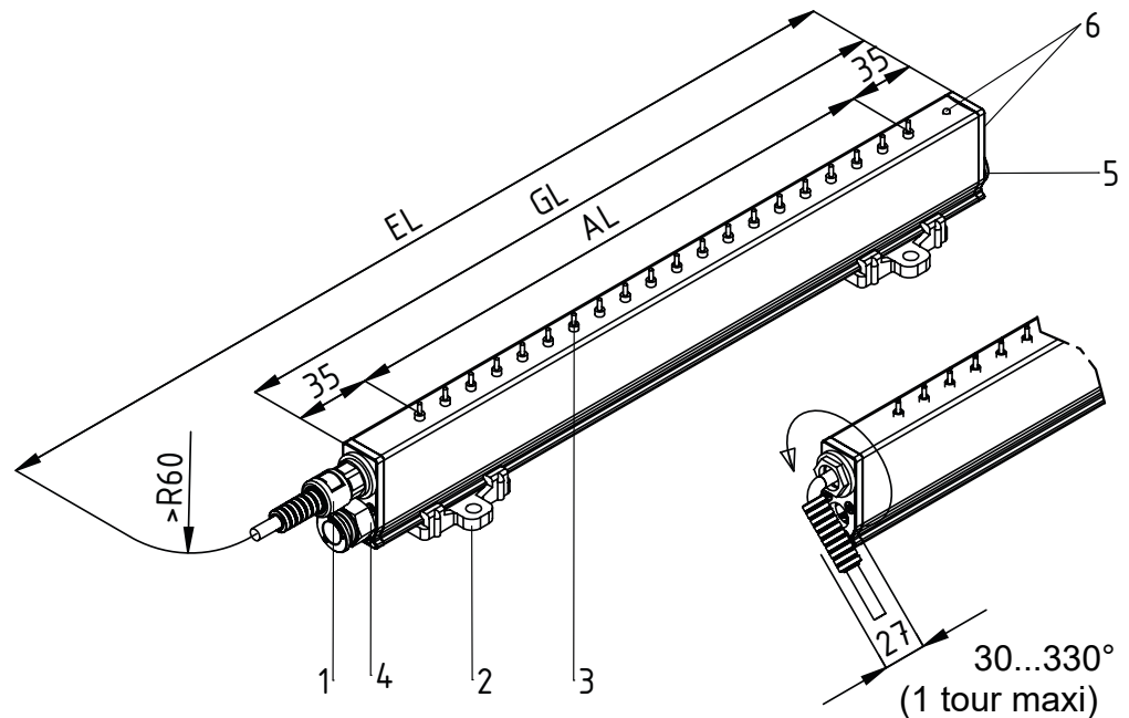
Fig. 1: Vue d'ensemble de l'électrode de décharge R60L
