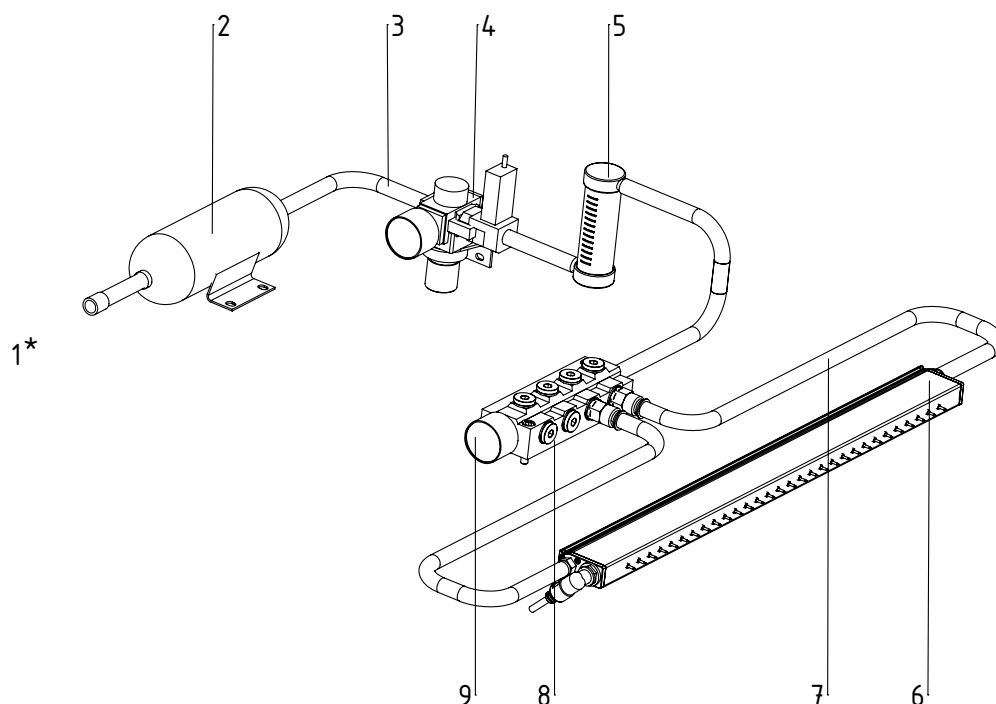
Fig. 9: Installation du système d'alimentation en air
