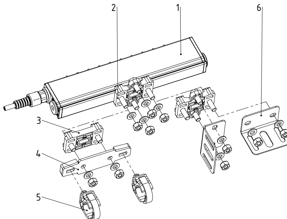
Fig. 2: Montage de l'électrode de décharge R60L
