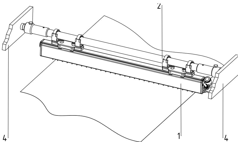
Fig. 4: Montage de l'électrode R60L avec la barre ronde en plastique renforcé par fibres de verre
