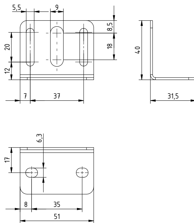
Fig. 15: Équiere de fixation
