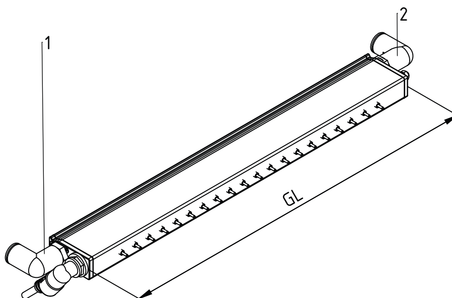
Fig. 8: Emplacement des raccords d'air en fonction de la lon- gueur totale GL
