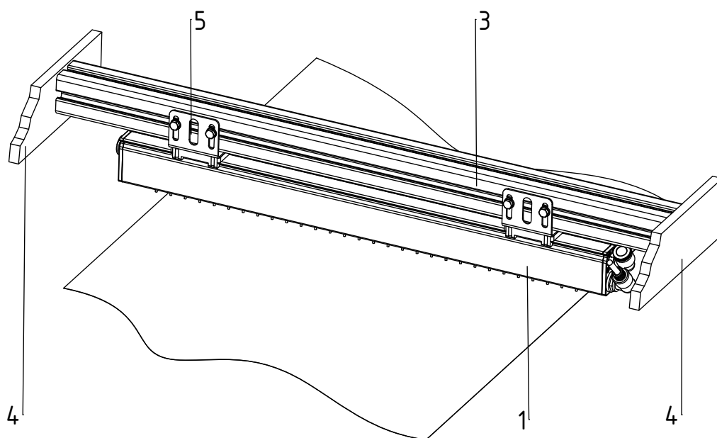
Fig. 3: Exemple de montage de l'électrode R60L avec une équerre en acier et un profilé en aluminium
