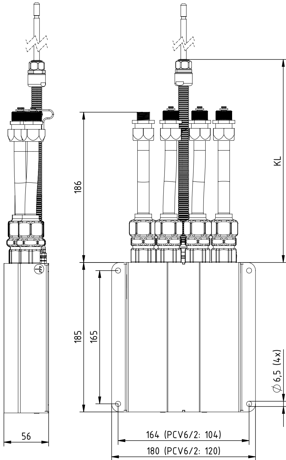
Fig. 7: Dimensions du distributeur PCV6/2, PCV6/4
