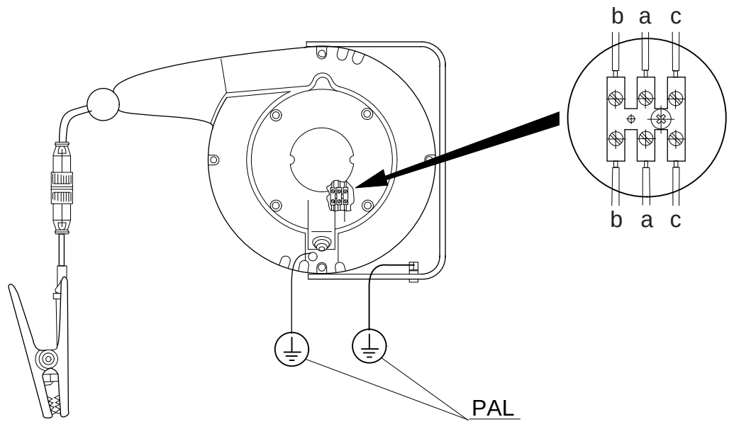
Fig. 6: Connexion de l'enrouleur de câ- ble 601KR/_
