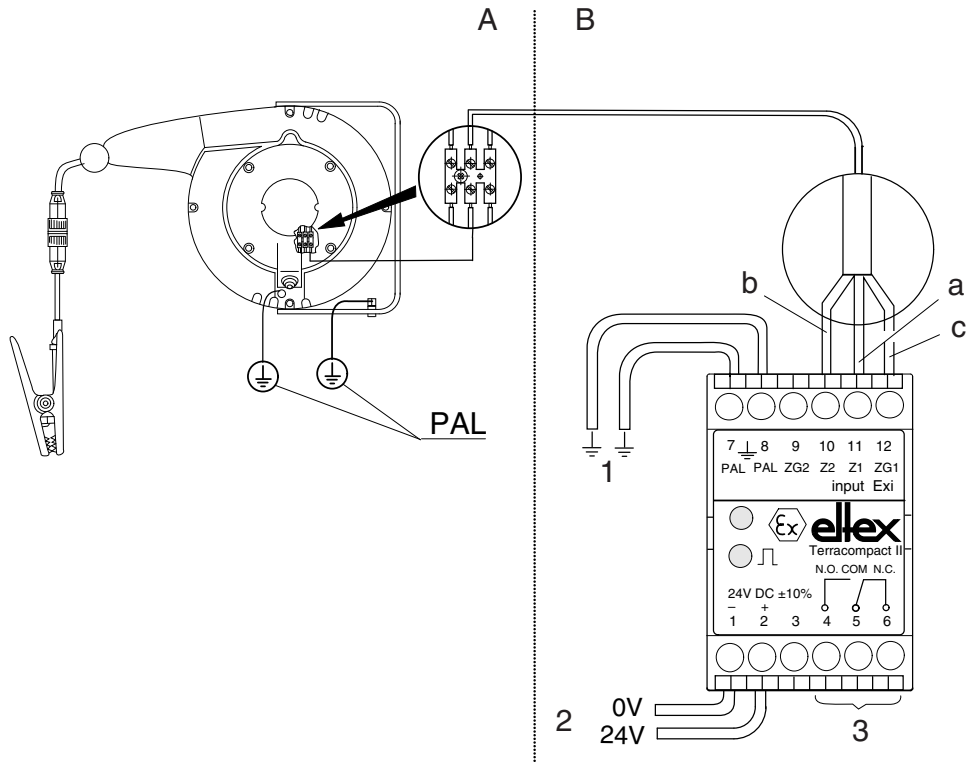
Fig. 10: Connexion électrique de l'enrouleur de câble automatique 601KR/_ au Terra-compact TCO030
