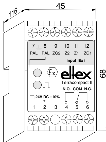
Fig. 15: Dimensions Terracompact II TCO030
