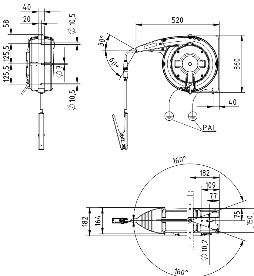
Fig. 2 : Montage de l'enrouleur de câble en aluminium Modèle 601KR/AW
