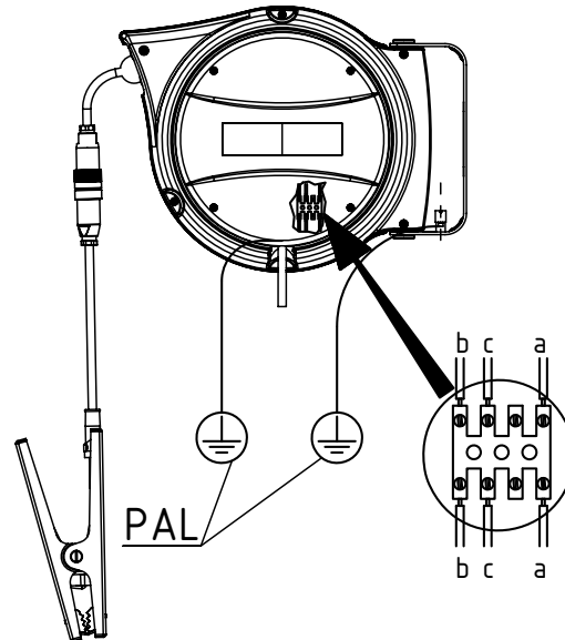
Fig. 10 : Connexion de l'enrouleur de câble en plastique 601KR/EW
