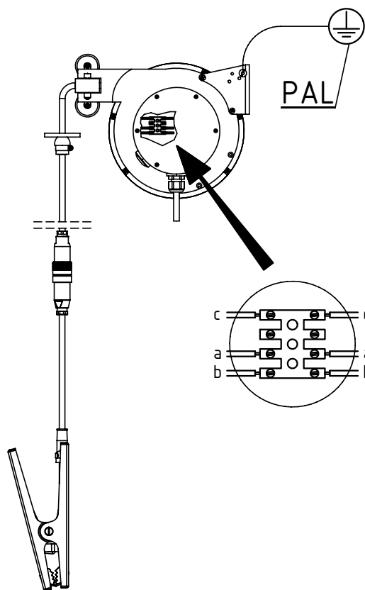
Fig. 9 : Connexion de l'enrouleur de câble en plastique 601KR/KW
