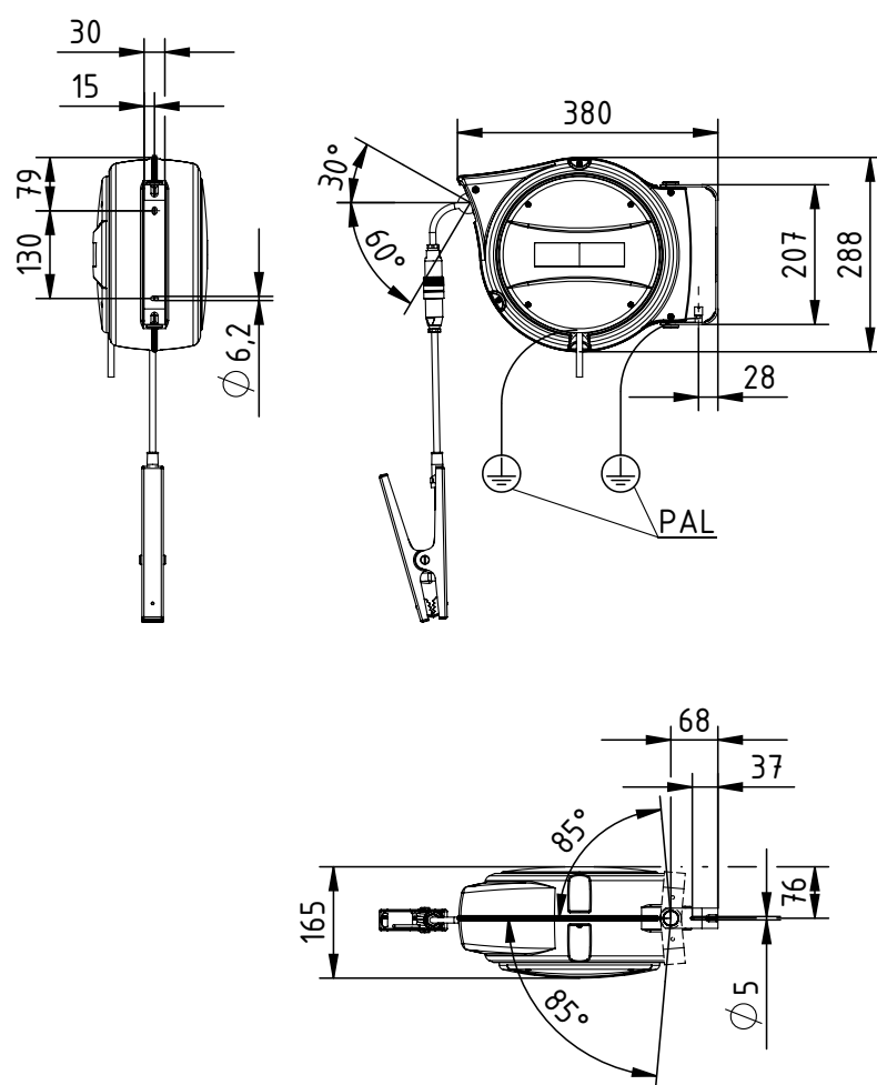
Fig. 3 : Montage de l'enrouleur de câble en aluminium Modèle 601KR/DW Modèle 601KR/EW
