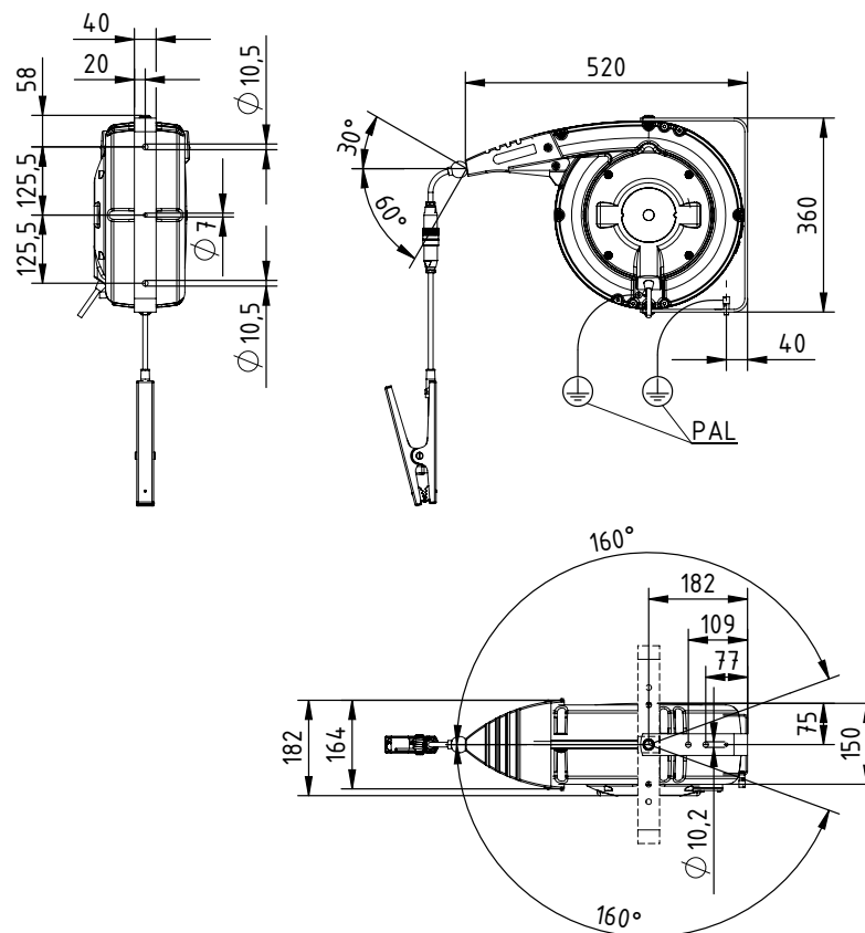
Fig. 12 : Enrouleur de câble en aluminium Modèle 601KR/AW
