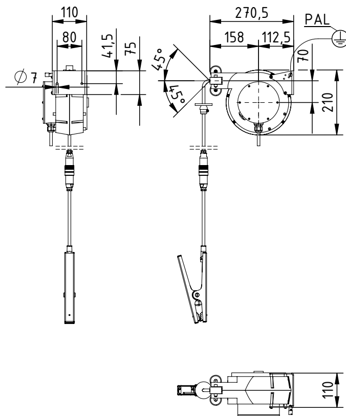
Fig. 6 : Montage de l'enrouleur de câ- ble en plastique Modèle 601KR/KW
