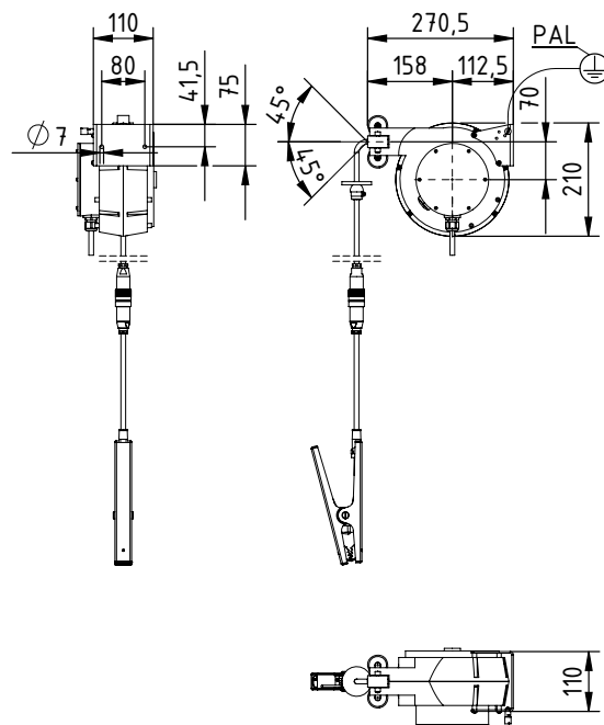
Fig. 28 : Enrouleur de câble automatique en aluminium Modèle 601KR/KW
