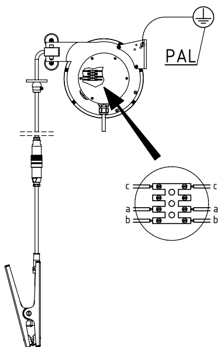
Fig. 11 : Connexion de l'enrouleur de câble automatique 601KR/KW
