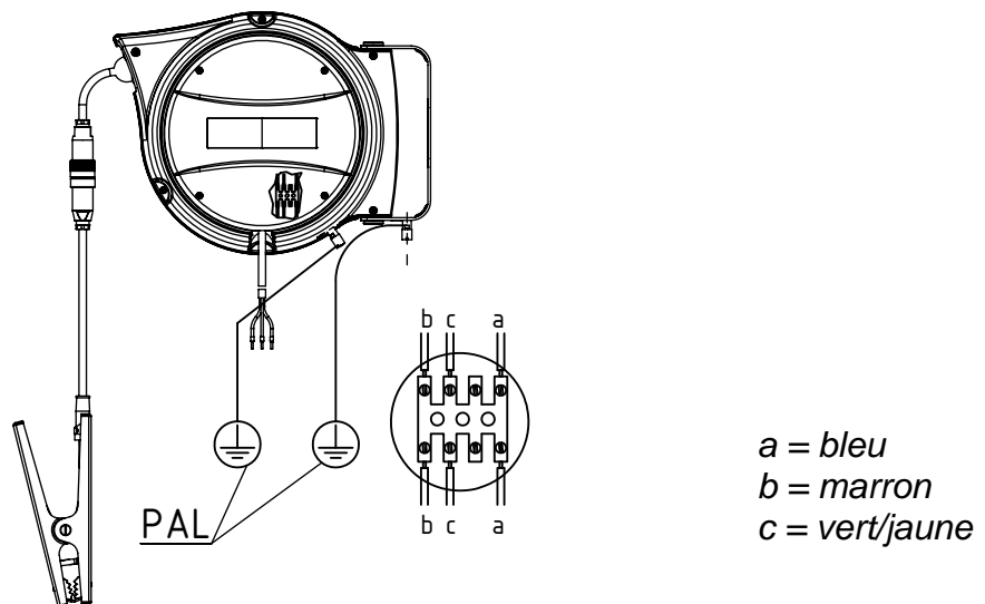
Fig. 10 : Connexion de l'enrouleur de câ- ble automatique 601KR/DW
