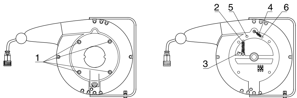
Fig. 15 : Dispositif d'arrêt de l'enrouleur de câble automa- tique en aluminium
