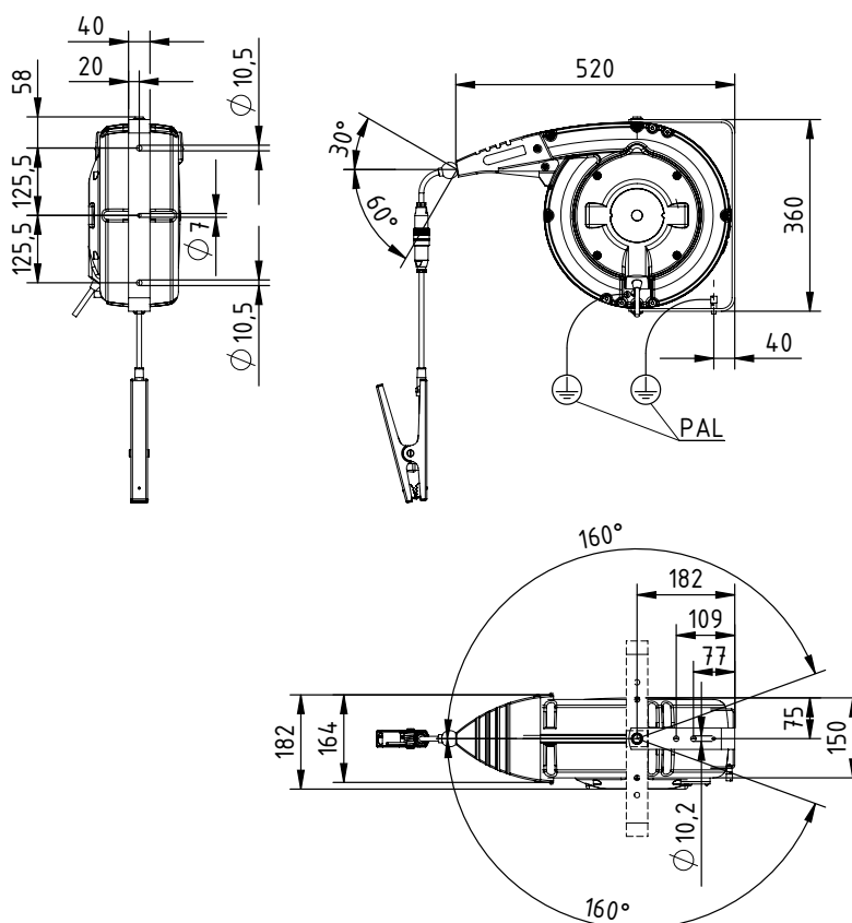
Fig. 26 : Enrouleur de câble automatique en aluminium Modèle 601KR/AW
