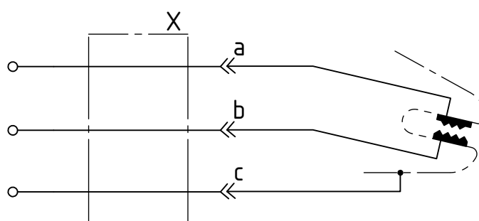
Fig. 13 : Schéma de connexion des pinces de mise à la terre modèles 70CG et 70CK avec câble et enrouleur de câble automatique
