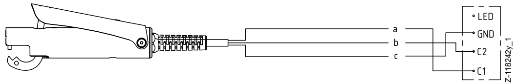
Fig. 11: Exemple de connexion d'un contacteur de mise à la terre TERRA-L
