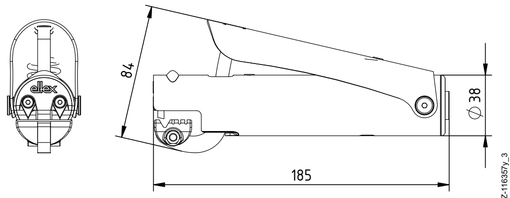
Fig. 10 : TERRA-C ouverture de pince maximale de 35 mm
