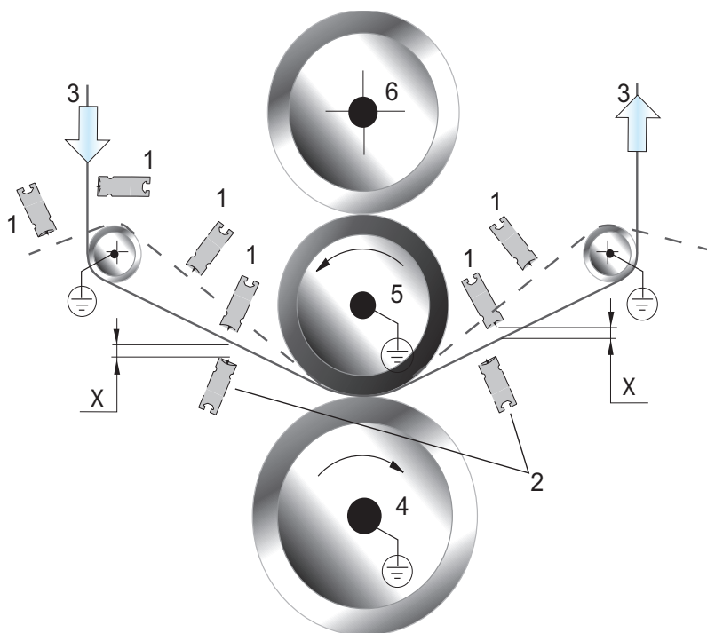
Fig. 12: Positionnement de l'électrode de décharge
