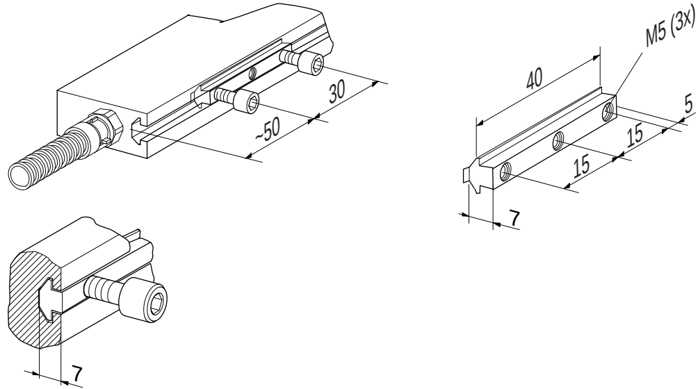
Fig. 11: Montage avec écrous coulissants
